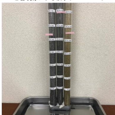
写真3 水の毛管水
