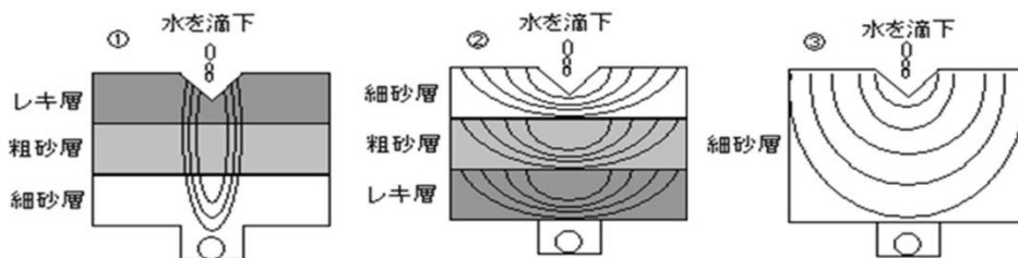
図4 水の縦移動
