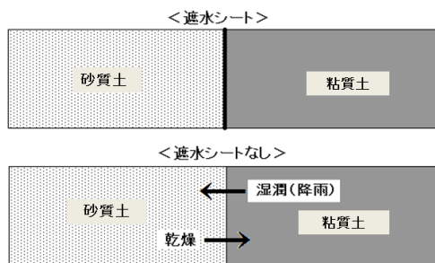
図3 水の横移動
