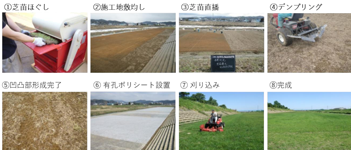
写真4 施工手順
